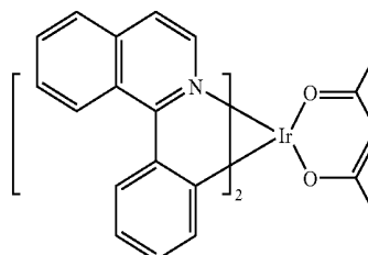
Ir(piq) 2 (acac)
