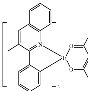
Ir(3-Mepq) 2 (acac)
